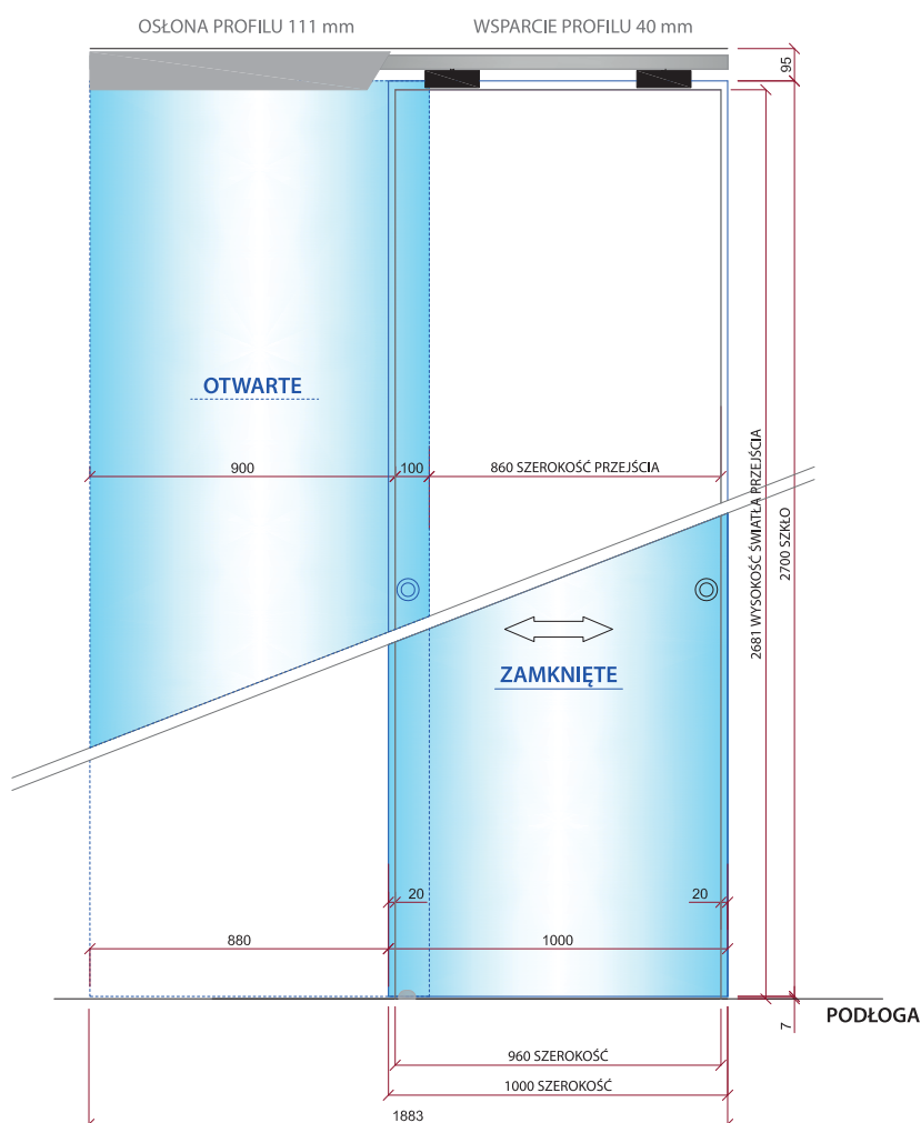
SYSTEM B DO MONTAŻU W NADPROŻU
